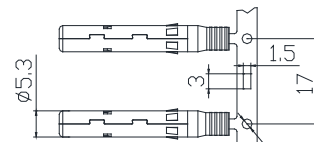
Contato do soquete fêmea (+)
