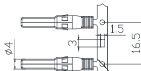
Contato do pino macho (-)
