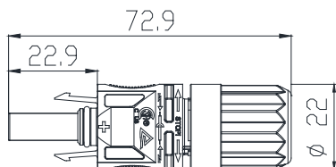
Conector Fêmea (+)
