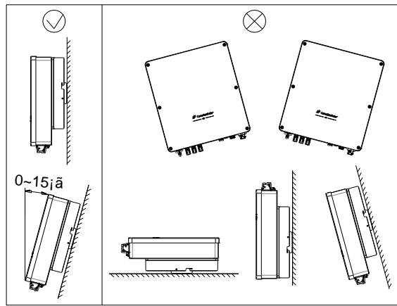
FIG.6-5 Requisitos de ângulo de instalação
