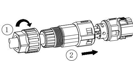
FIG.6 Montagem do conector
