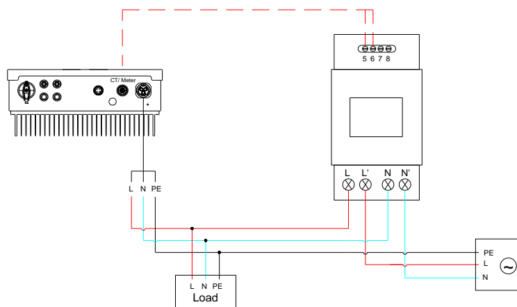
FIG.2 Diagrama de conexão eléctrica e de sinal
