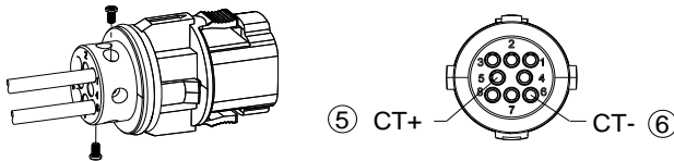
FIG.5 As posições dos pinos do conector
