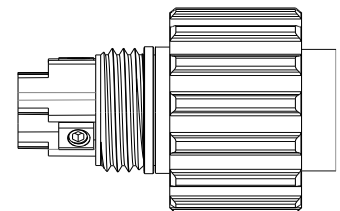
Plugue (pinos de metal e carcaça)
