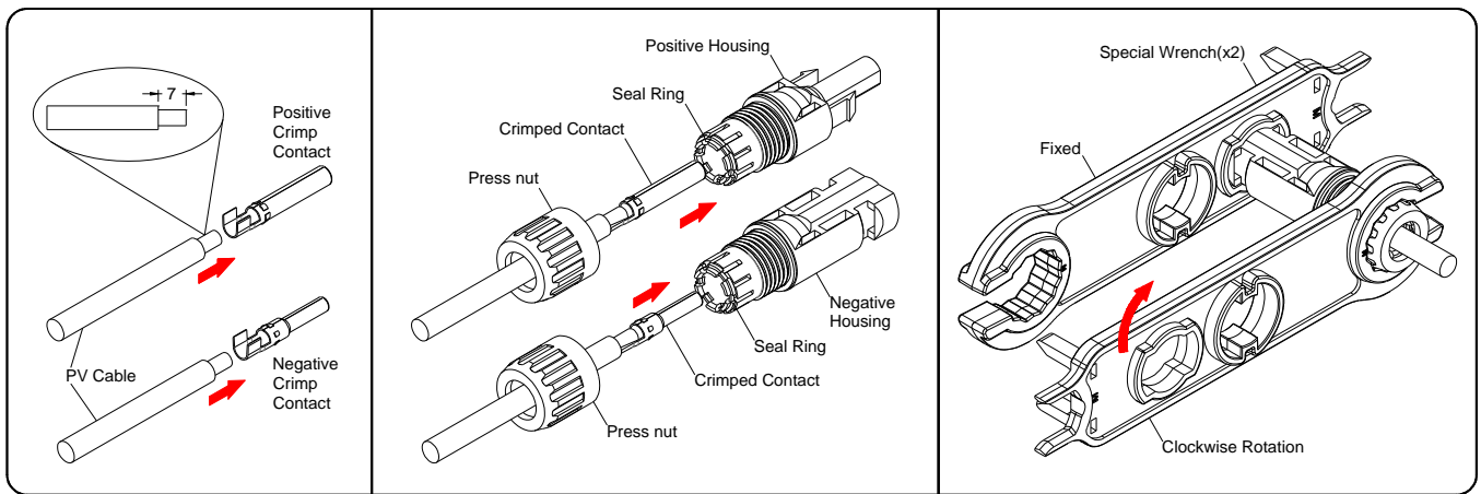
FIG.7-9 Cabeamento de entrada CC
