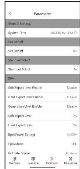
FIG.10 Configuração na página EPM
