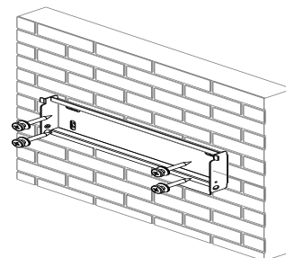
FIG.6-8 Fixe o suporte de montagem na parede
